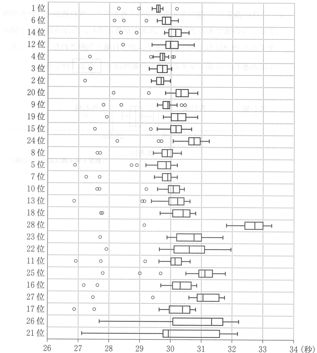
図 3 28 人の選手の順位と 30 個のタイムの箱ひげ図(上から分散の小さい順)
